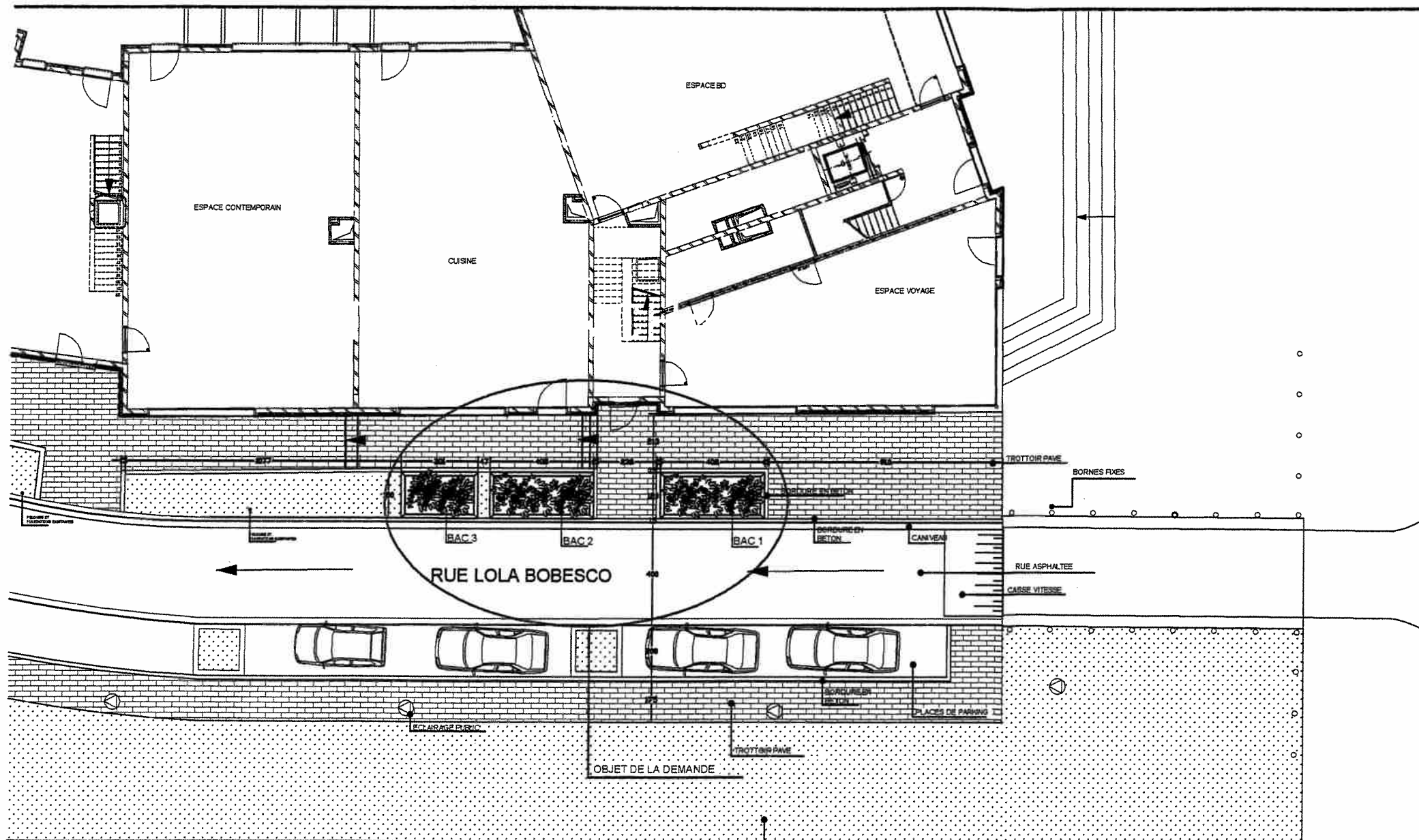
VUE EN PLAN - SITUATION PROJETEE
